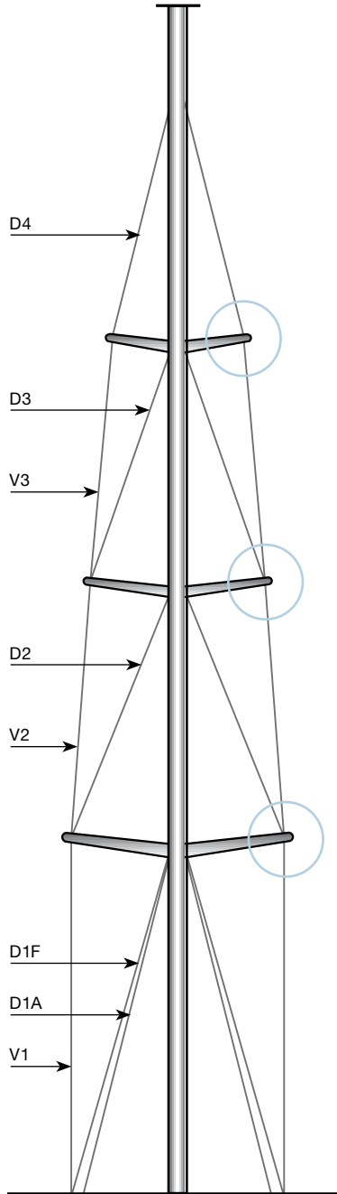
Gelinktes Mittelwant.
