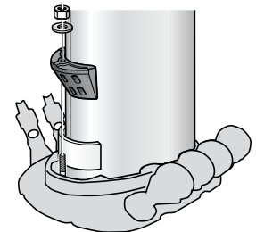
Stellen des Mastes und Einsetzen des Keiles.
