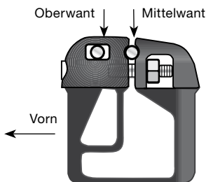
Salingendbeschlag zum Einklemmen für durchgehendes Mittelwant.
