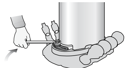
Sichern und Einspannen des Mastes durch Anziehen der Mutter.
