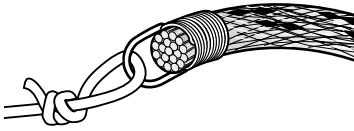
Takling mit Auge.
