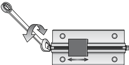
Verstellbarer T-Beschlag. Entspannen Sie das stehende Gut und verstellen Sie den Mastfuß bei stehendem Mast.
