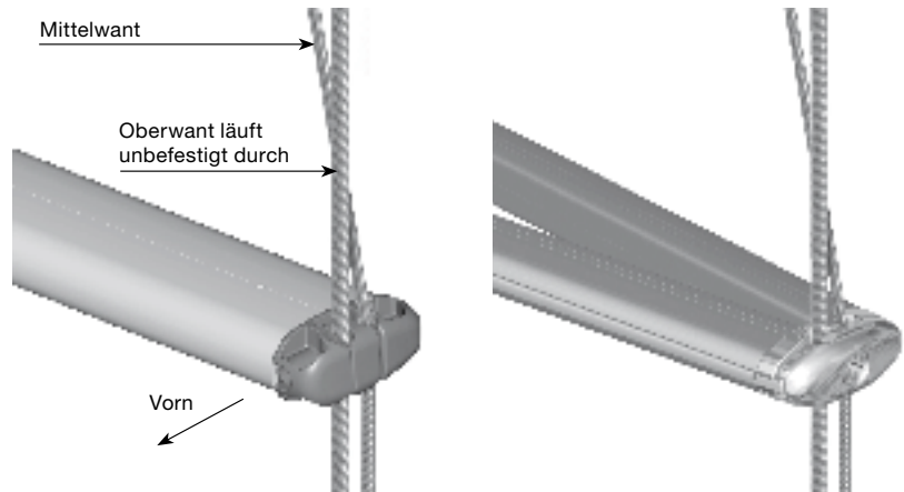
Salingendbeschlag für durchgehende Mittelwanten.
