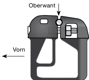
Salingendbeschlag zum Einklemmen des Oberwants bei Ein-Saling-Riggs und für Mittelwant bei Mehrsaling-Riggs.
